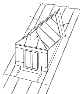
Helbeslagen kupa
